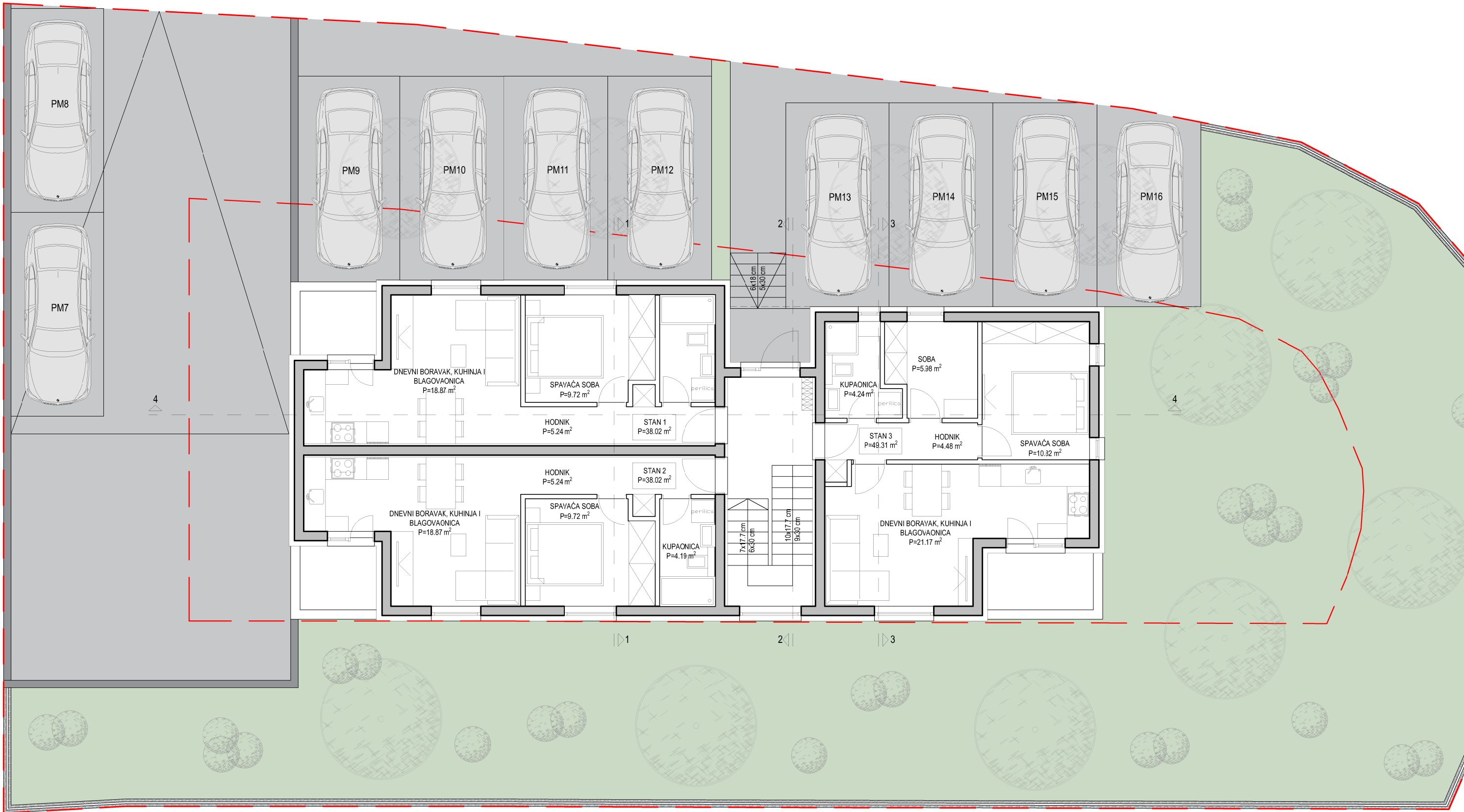
TLOCRT PRIZEMLJA M 1:100
